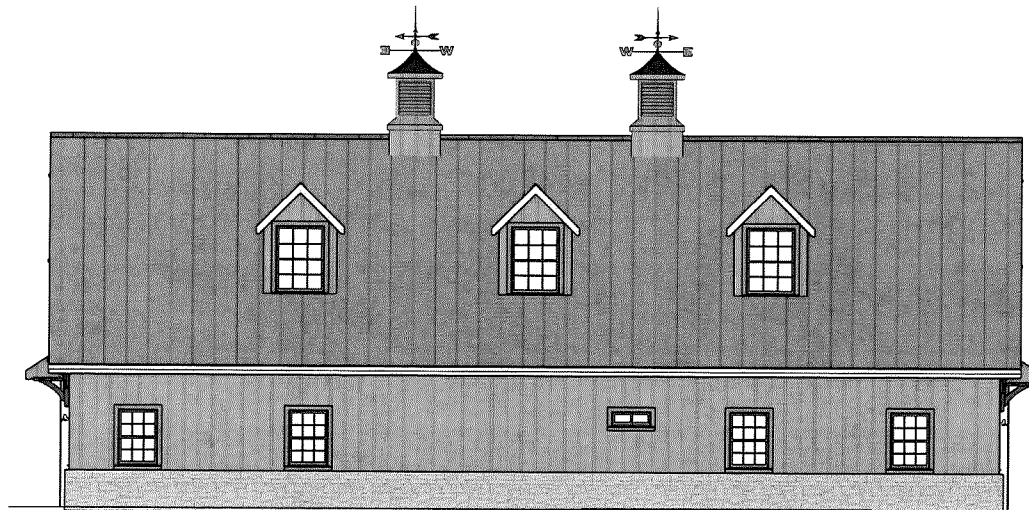
E4 ELEVATION SCALE: 1/4" = 1'-0"
