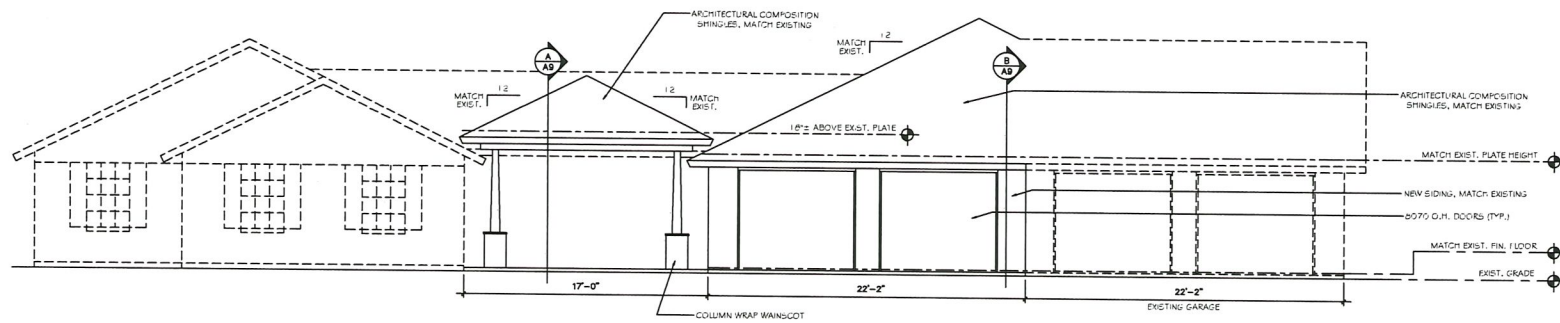
A A4 EAST EXTERIOR ELEVATION SCALE: 1/4"=1'-0"
