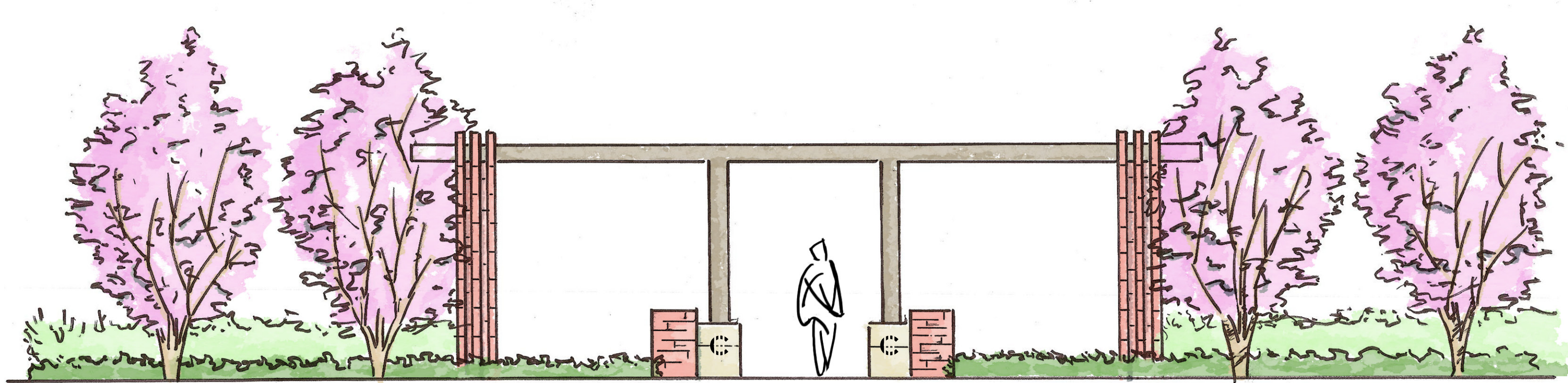
ELEVATION A-A' 0' 1' 2' 4' 8' SCALE: 1/4"=1'-0"
